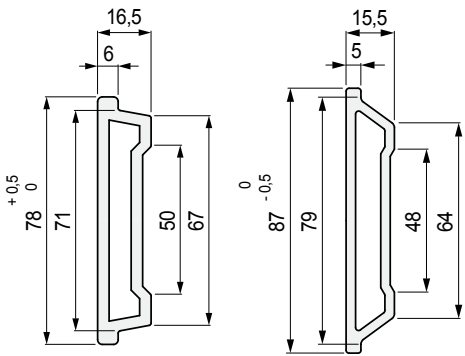
Part. S0191
